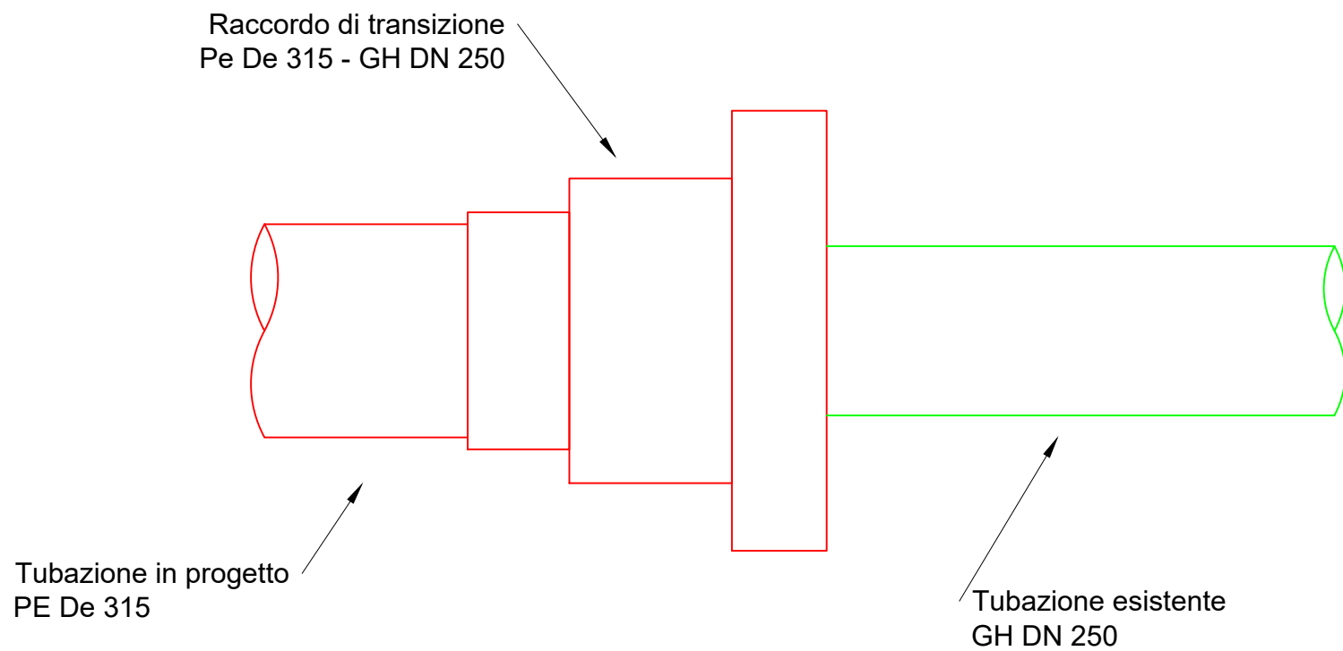
Tipologico 14 Raccordo di Transizione Pe De 315 - GH DN 250 Nodi 22
