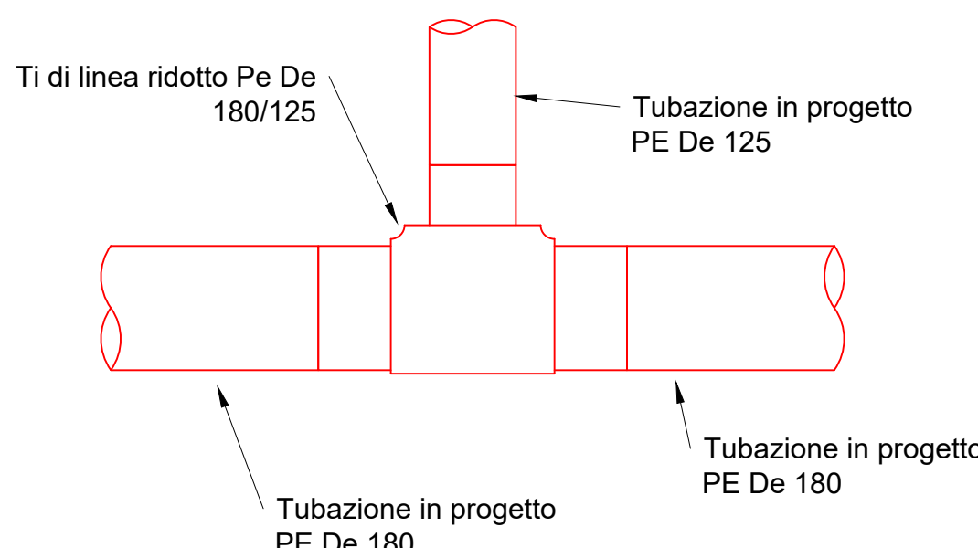
Tipologico 29 Ti in linea ridotto Pe De 180 - Pe De 125 Nodi 44-84
