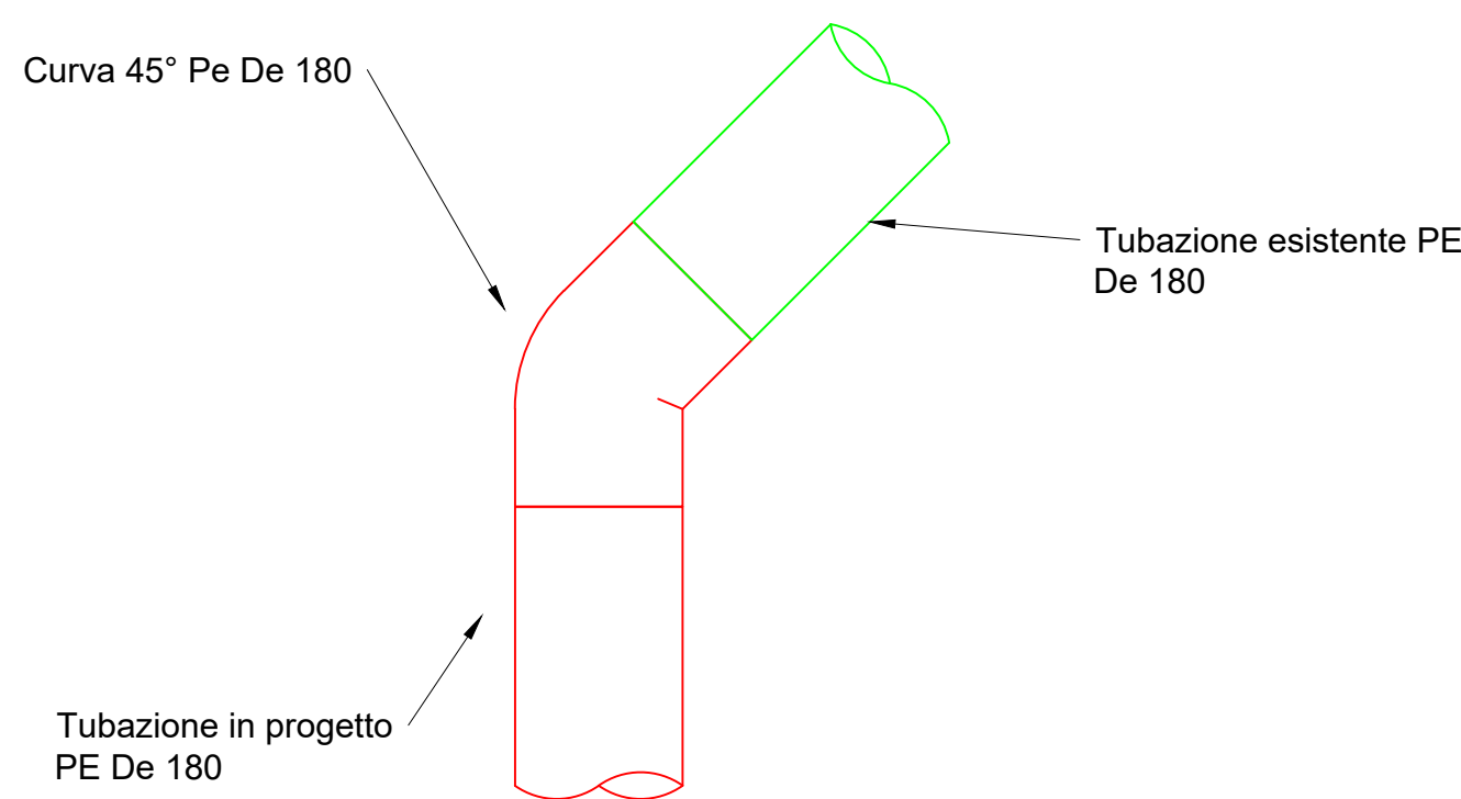
Tipologico 2 Collegamento in linea curva 45° Pe De 180 Nodo 1-18-38-43-54-63-64-68-80-107
