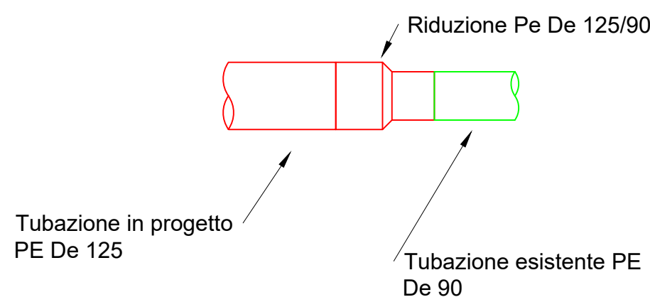
Tipologico 17 Riduzione Pe De 125 - Pe De 90 Nodi 20
