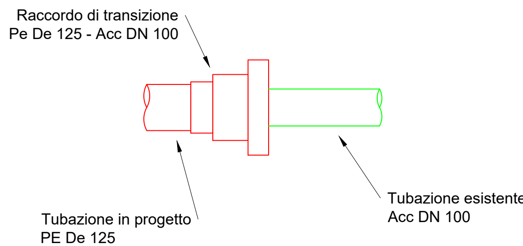
Tipologico 9 Raccordo di Transizione Pe De 125 - Acc DN 100 Nodi 119-32
