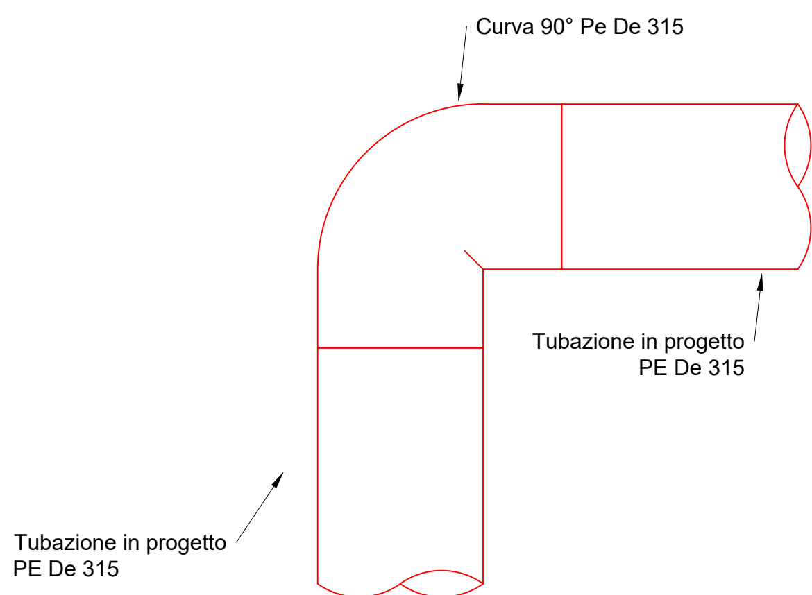
Tipologico 5 Curva 90° Pe De 315 Nodi 41
