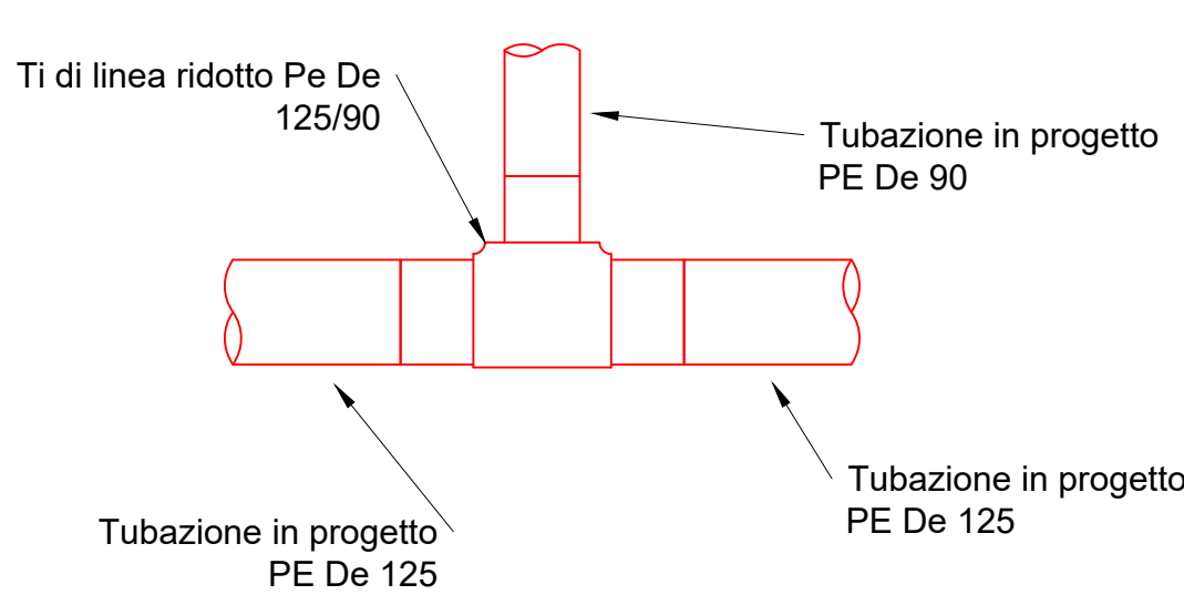
Tipologico 28 Ti in linea ridotto Pe De 125 - Pe De 90 Nodi 23-33-45
