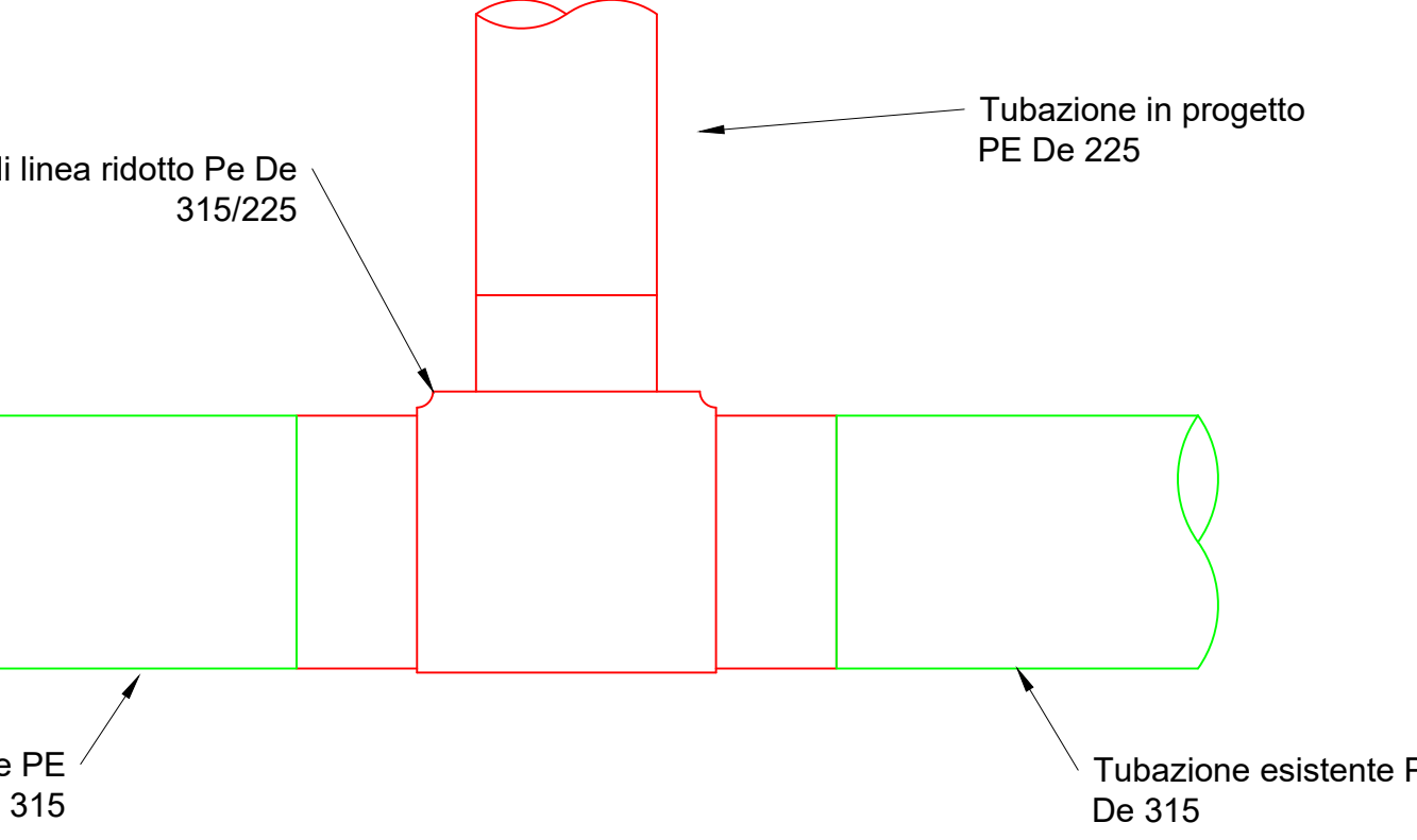
Tipologico 33 Ti in linea ridotto Pe De 315/225 Nodi 24-26-70-82-83-88-91-93-94-95-96- 97-98-100-102-103-104-105-121-123
