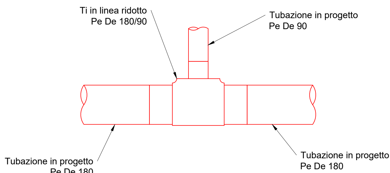
Tipologico 30 Ti in linea ridotto Pe De 180 - Pe De 90 Nodi 10-11-12-13-14-39-40-52-53-57-60-61- 62-86-108-109-110-111-114-115
