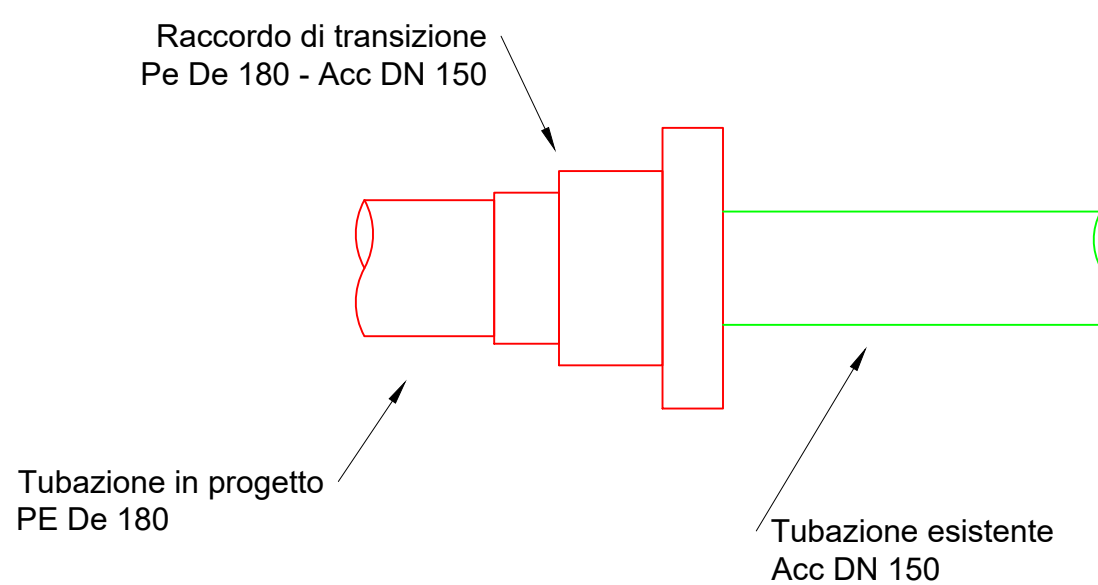
Tipologico 11 Raccordo di Transizione Pe De 180 - Acc DN 150 Nodi 16-51- 59-87-90-92-99-113-116-122
