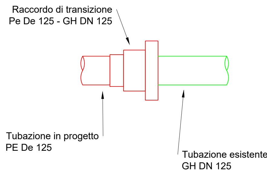
Tipologico 10 Raccordo di Transizione Pe De 125 - GH DN 125 Nodi 8
