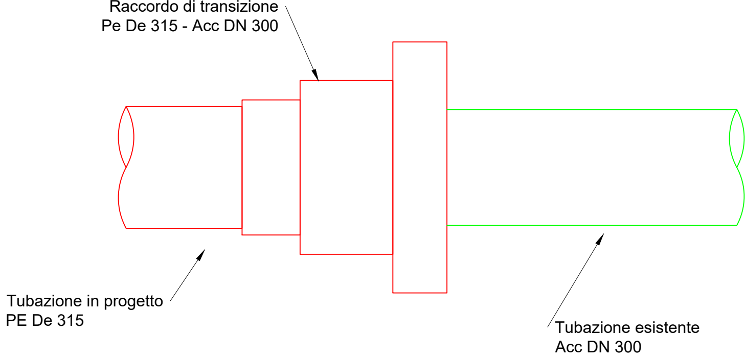
Tipologico 13 Raccordo di Transizione Pe De 315 - Acc DN 300 Nodi 2-77-118
