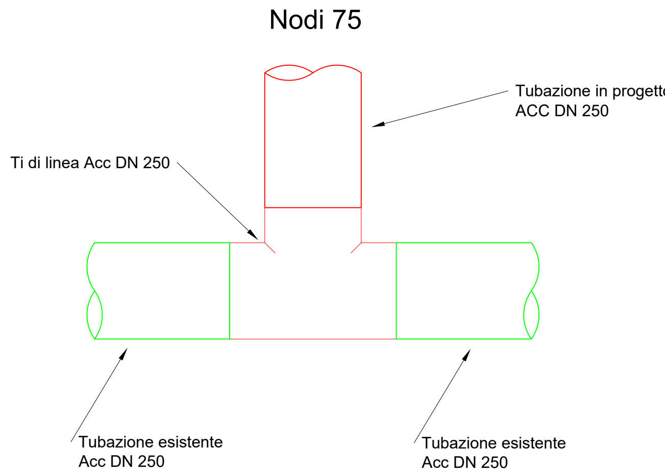
Tipologico 20 Ti di linea ACC DN 250
