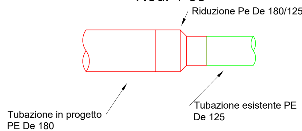
Tipologico 18 Riduzione Pe De 180 - Pe De 125 Nodi 4-65
