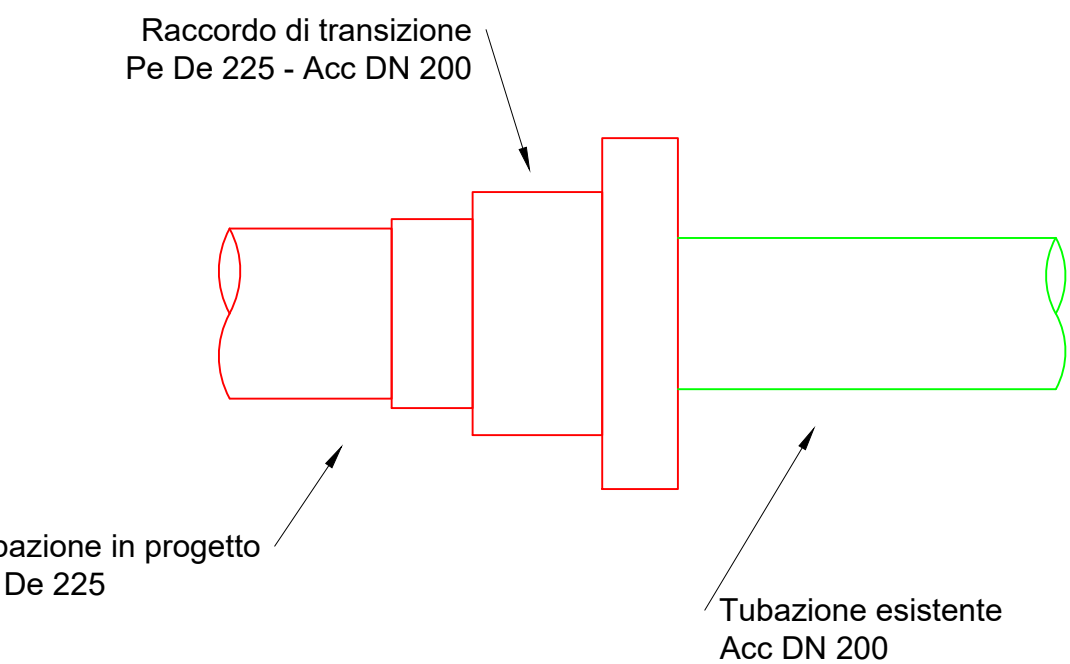
Tipologico 12 Raccordo di Transizione Pe De 225 - Acc DN 200 Nodi 36-42
