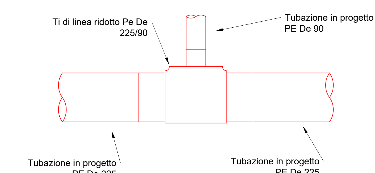
Tipologico 32 Ti in linea ridotto Pe De 225/90 Nodi 71-72
