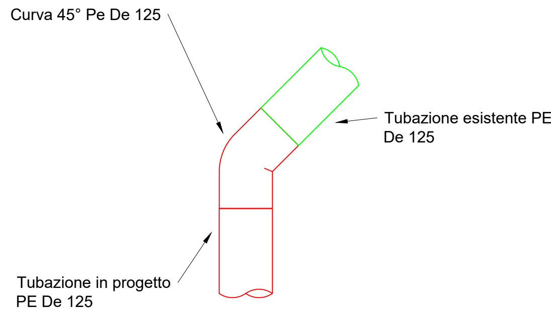
Tipologico 1 Collegamento in linea curva 45° Pe De 125 Nodi 66-85
