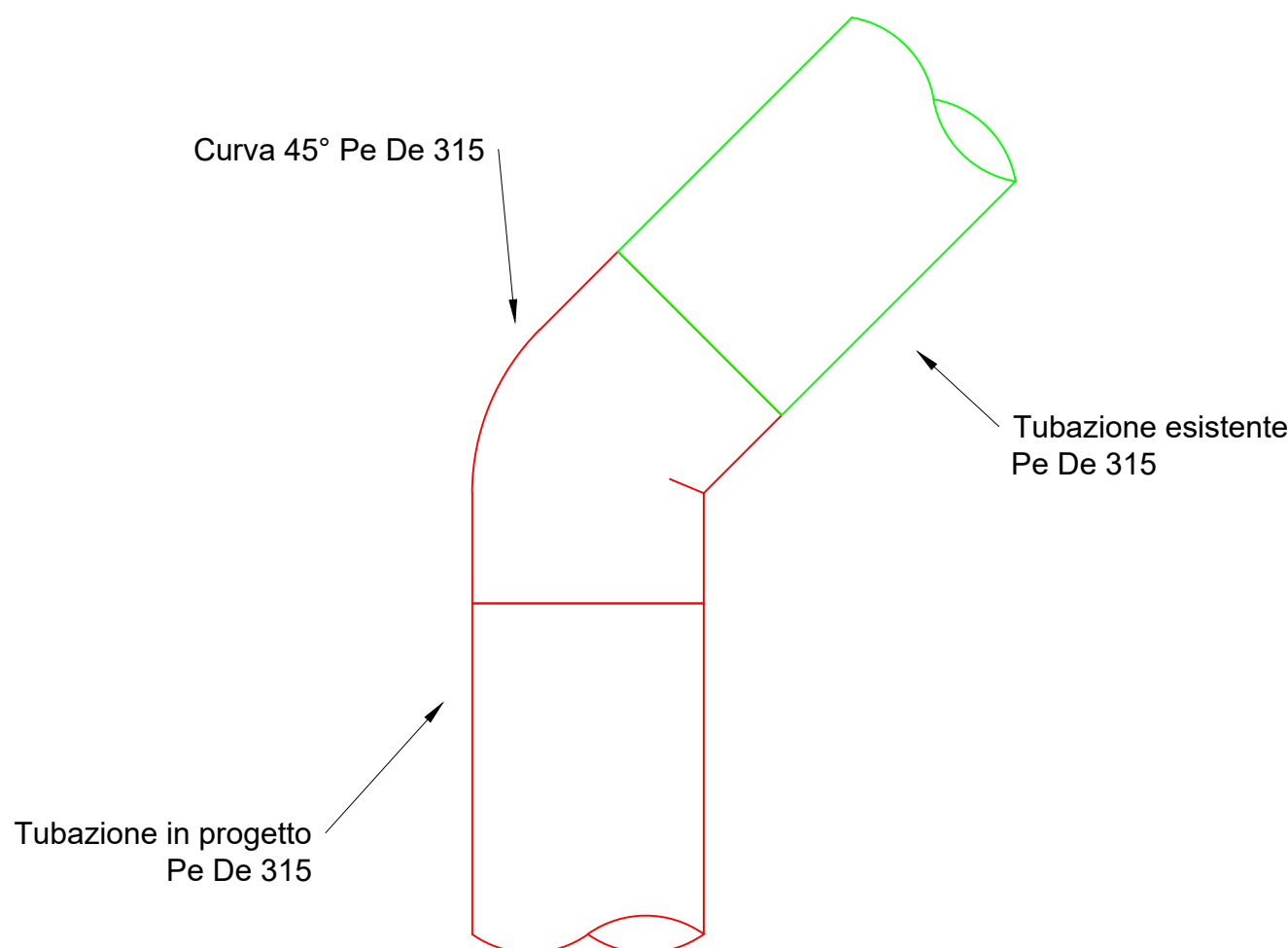
Tipologico 3 Collegamento in linea curva 45° Pe De 315 Nodi 106
