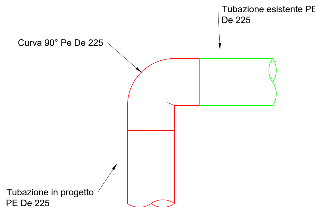
Tipologico 4 Curva 90° Pe De 225 Nodo 25
