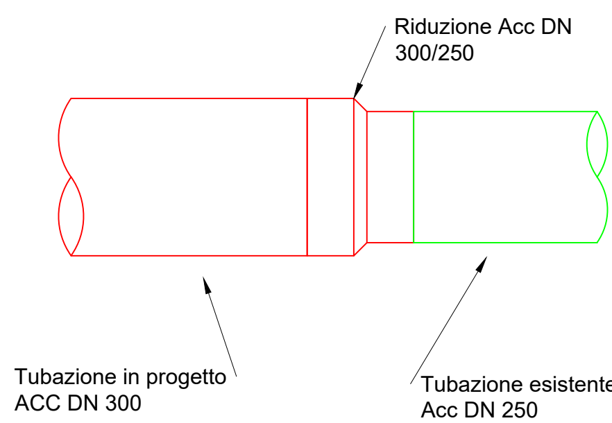
Tipologico 15 Riduzione ACC DN 300 - ACC DN 250 Nodi 81
