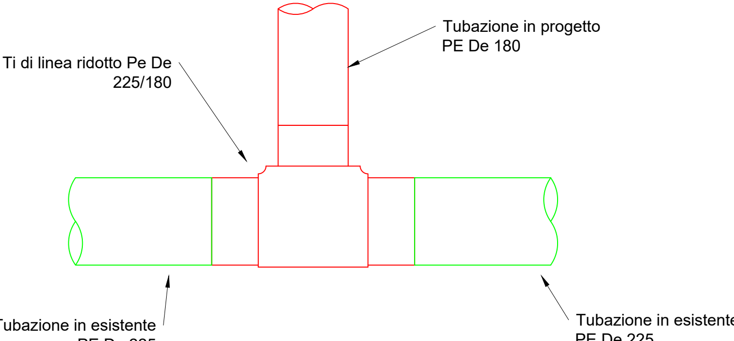
Tipologico 31 Ti in linea ridotto Pe De 225 - Pe De 180 Nodi 58
