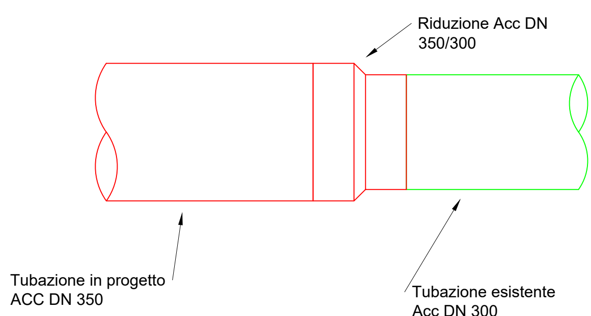
Tipologico 16 Riduzione ACC DN 350 - ACC DN 300 Nodi 79
